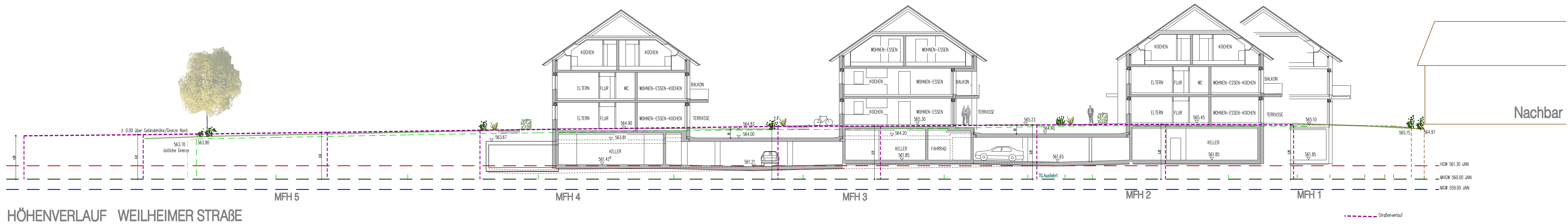
4 MEHRFAMILIENHÄUSER UND 11 REIHENHÄUSER SCHNITTE MEHRFAMILIENHÄUSER
