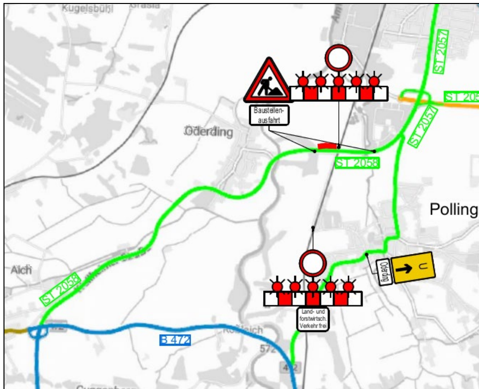
Lageplan Sperrung/Umleitung nördlicher Zubringer St2058 KFZ
