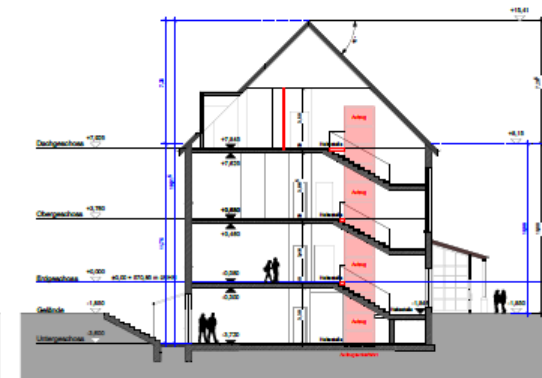
Schnitt A-A 1:100
