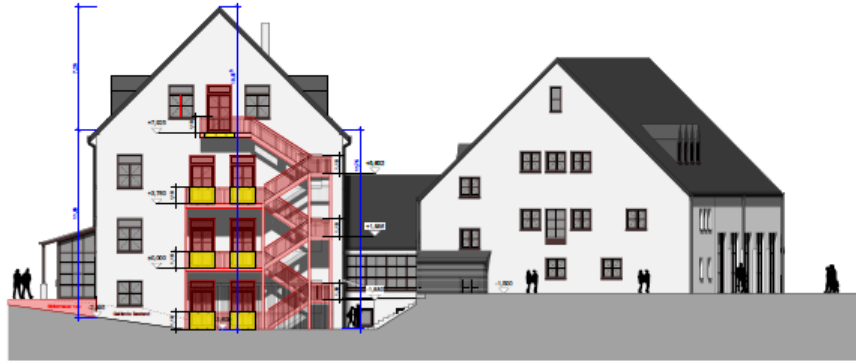
Ansicht West 1:100
